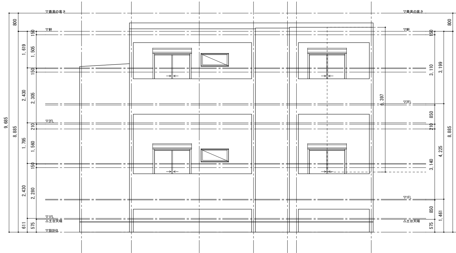
南立面図
