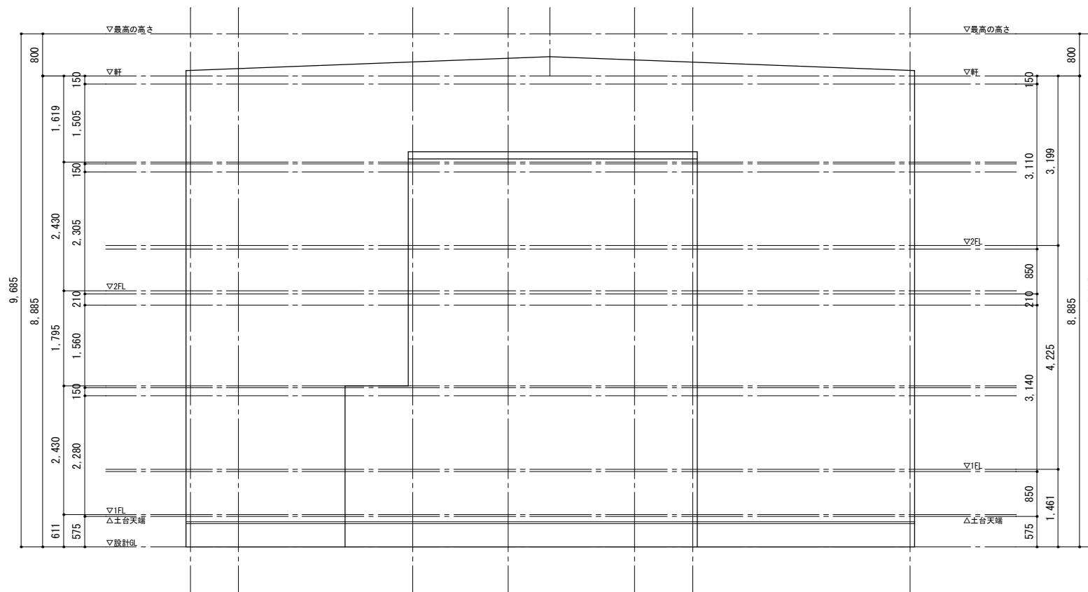
西立面図
