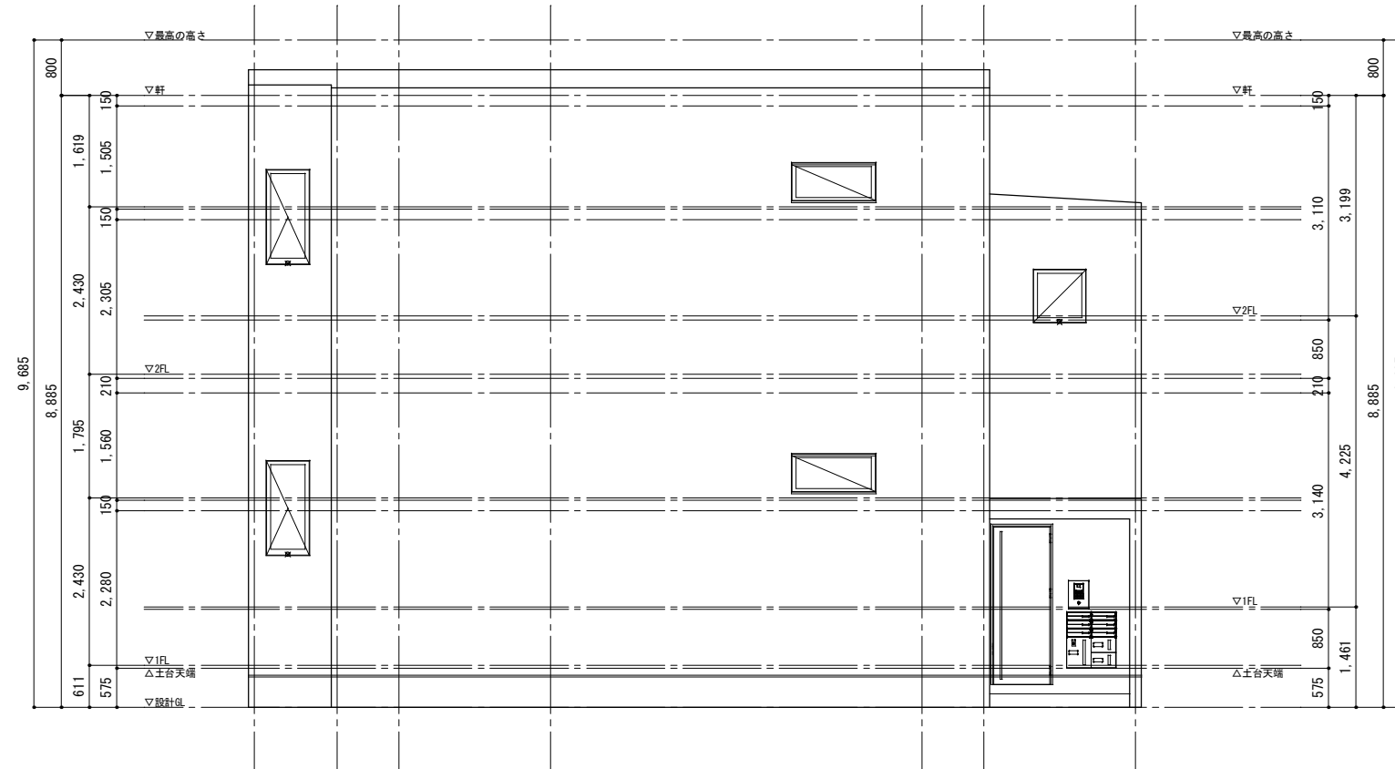
北立面図
