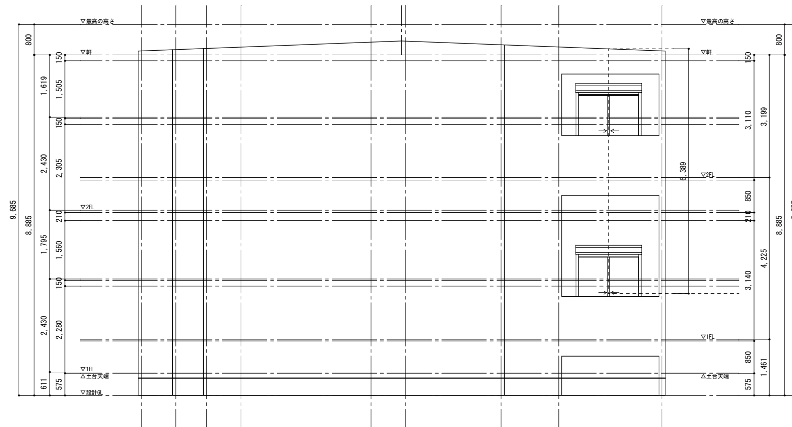
東立面図
